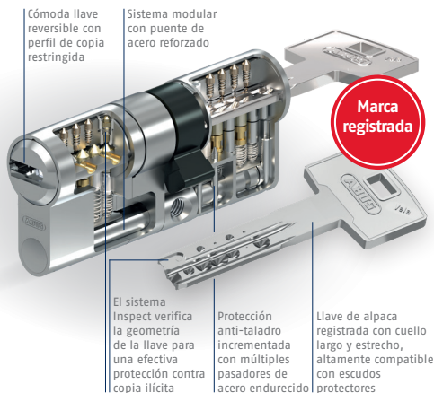
Detector Inspect en el rotor
