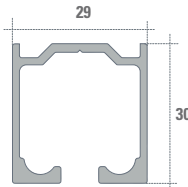
RIEL U45 RECTO TRACK U45 FLAT
